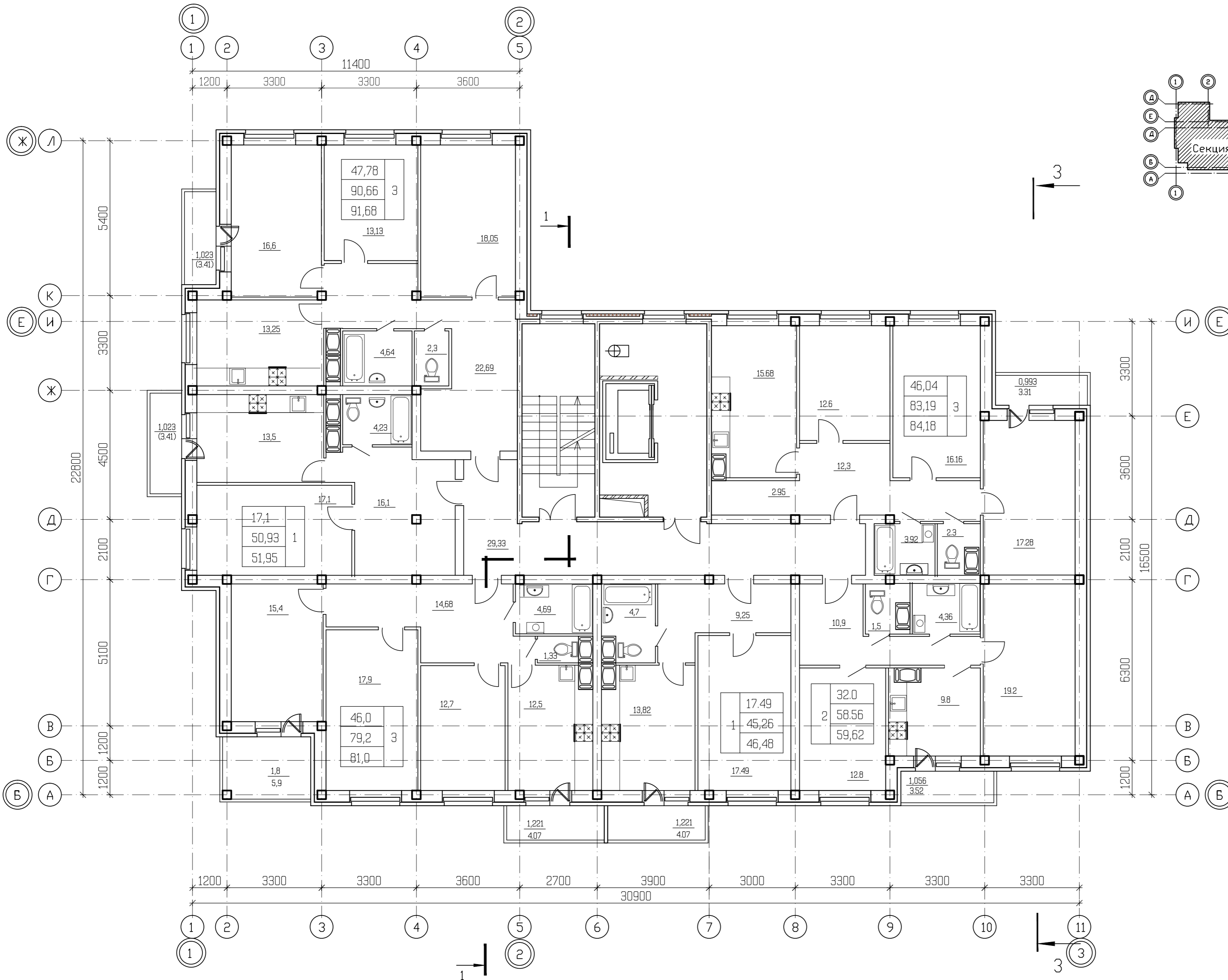
Компоновочная схема жилого дома №53
